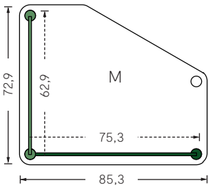
FLEX TABLE Fünfecktisch M
