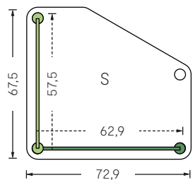
FLEX TABLE Fünfecktisch S
