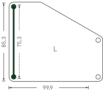
FLEX TABLE Fünfecktisch L
